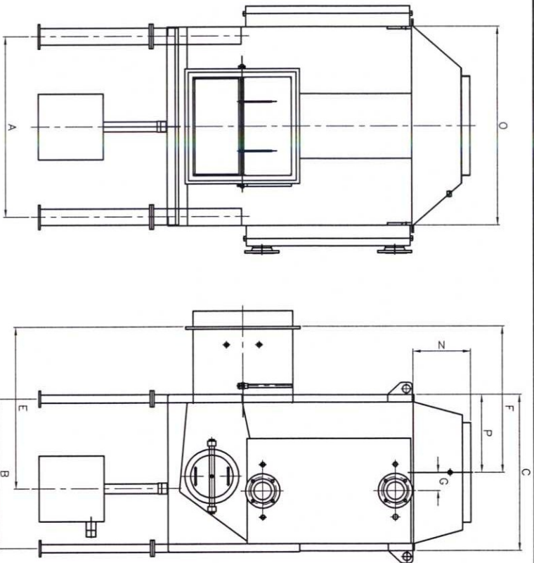
Vooranzicht
