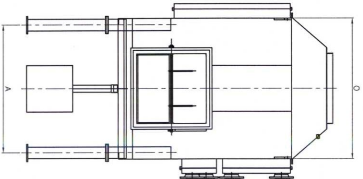
Vooraanzicht
